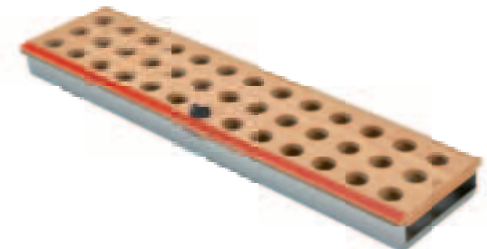
Collet holder ER 25 complete
